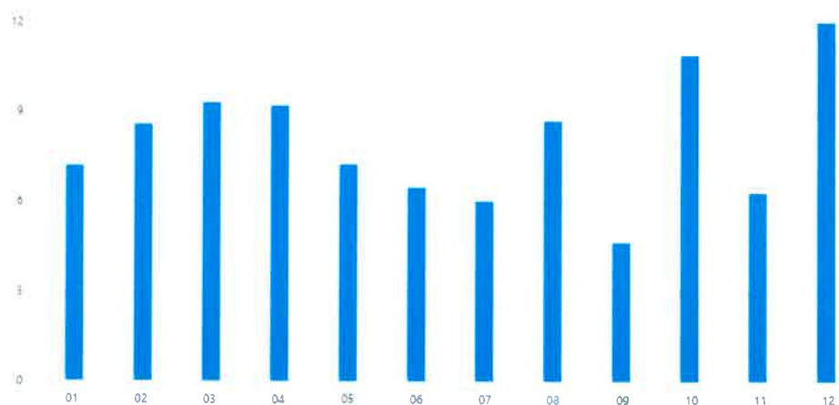
Produkce odpadů
